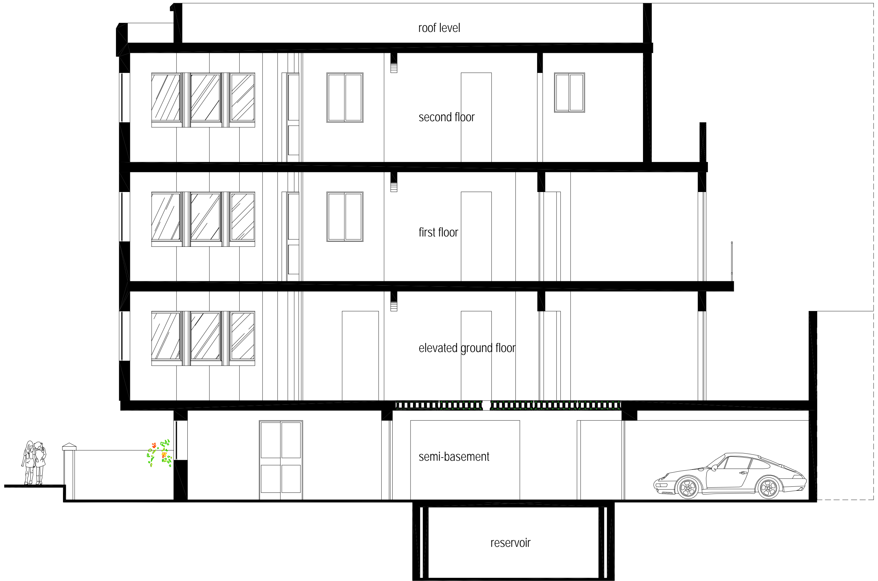
Longitudinal Section A-A
